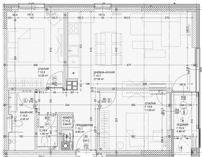
Г АП 15 81.41 кв.м.
